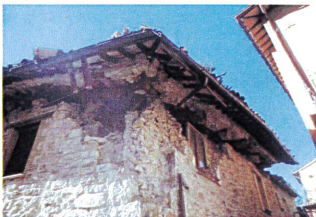
Figura 21 Comportamento di tetto con orditura a puntoni lignei a spinta non compensata. Visso (MC).
